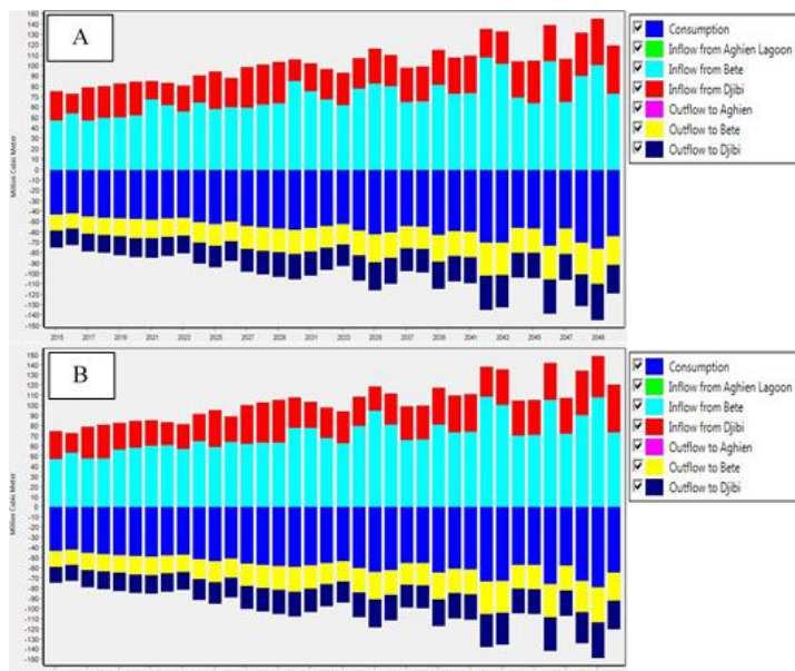
Fig. 9; The flows of demand sites in 2050 for the scenarios « SR » (A) and « SC » (B).
